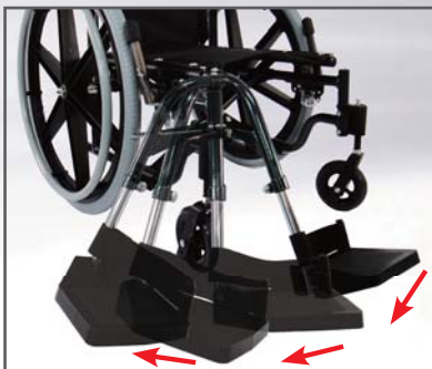
スイングアウト式ハンガー およびフットプレート
