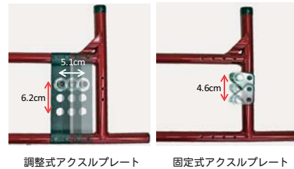
調整式アクスルプレート 固定式アクスルプレート
